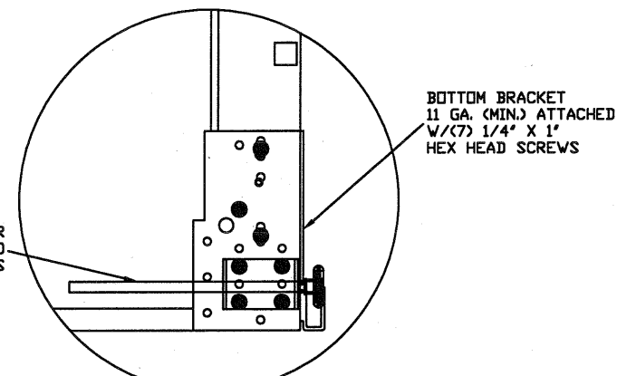
TYPICAL BOTTOM BRACKET N.T.S.
