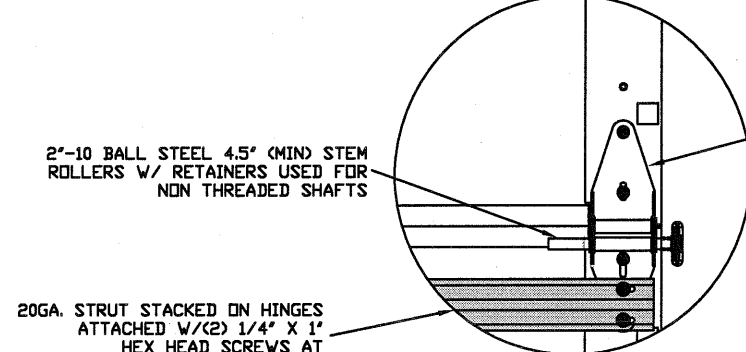
TYPICAL END HINGE N.T.S.
